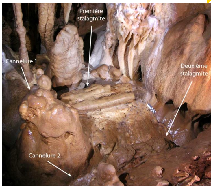
Figure 9. Deux stalagmites de dérivation. La première est située en haut (couleur blanche) et la deuxième un peu plus bas dans le creux (couleur marron).
