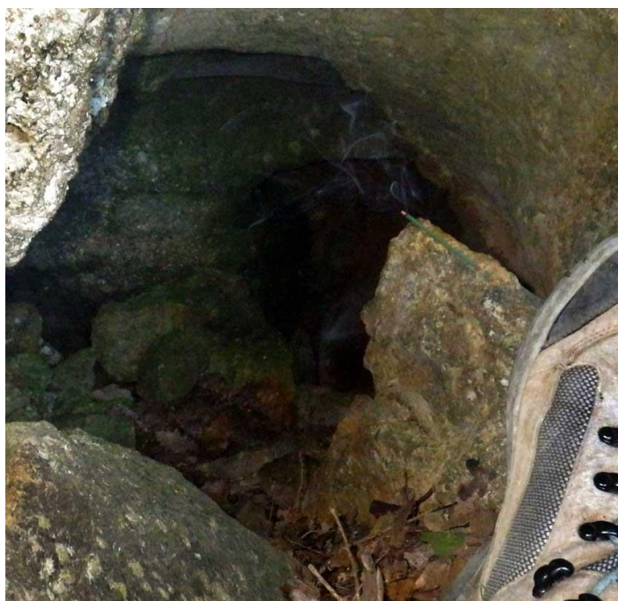
Figure 2. L'entrée de la grotte du Serre des Périers le jour de sa découverte (28 janvier 2018). La fumée du bâton d'encens est aspirée par le trou. La chaussure à droite donne l'échelle.
