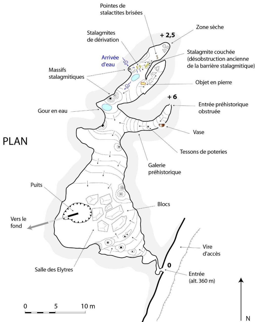
Fig. 15 : Plan de la partie préhistorique de la grotte : salle des Elytres et ses prolongements.
